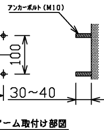
アーム取付け部図
