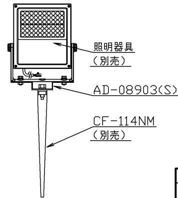
組立図
