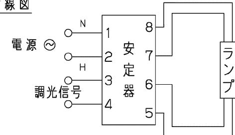
結線図
