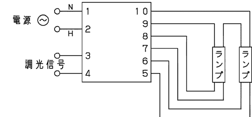
結線図
