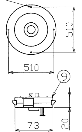
4-φ4.5木ねじ用K,O
