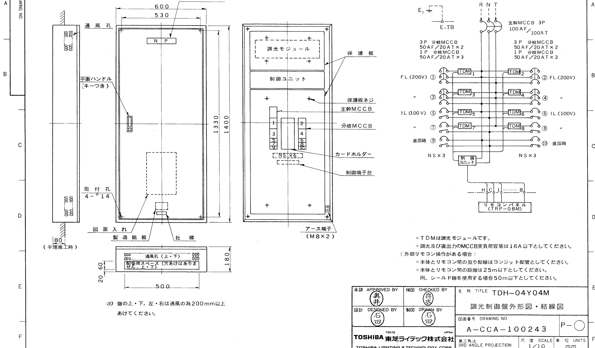
外形図
