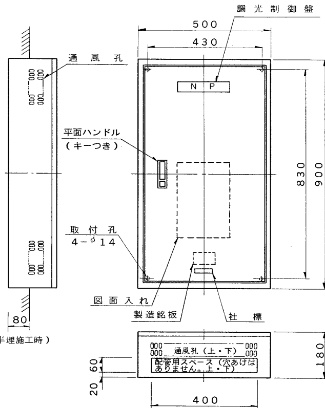
外形図
