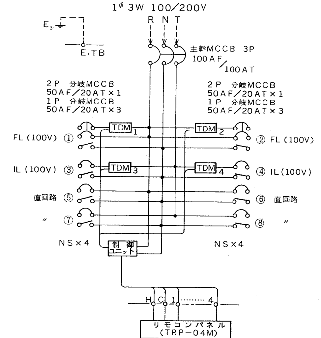
結線図
