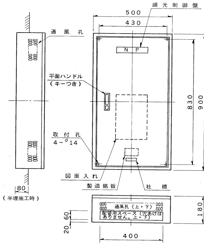
外形図
