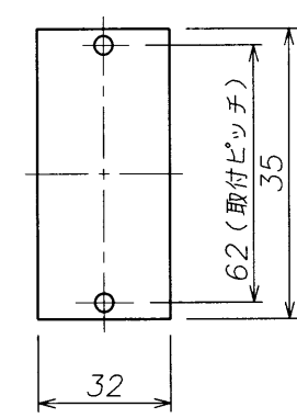
取付寸法図
