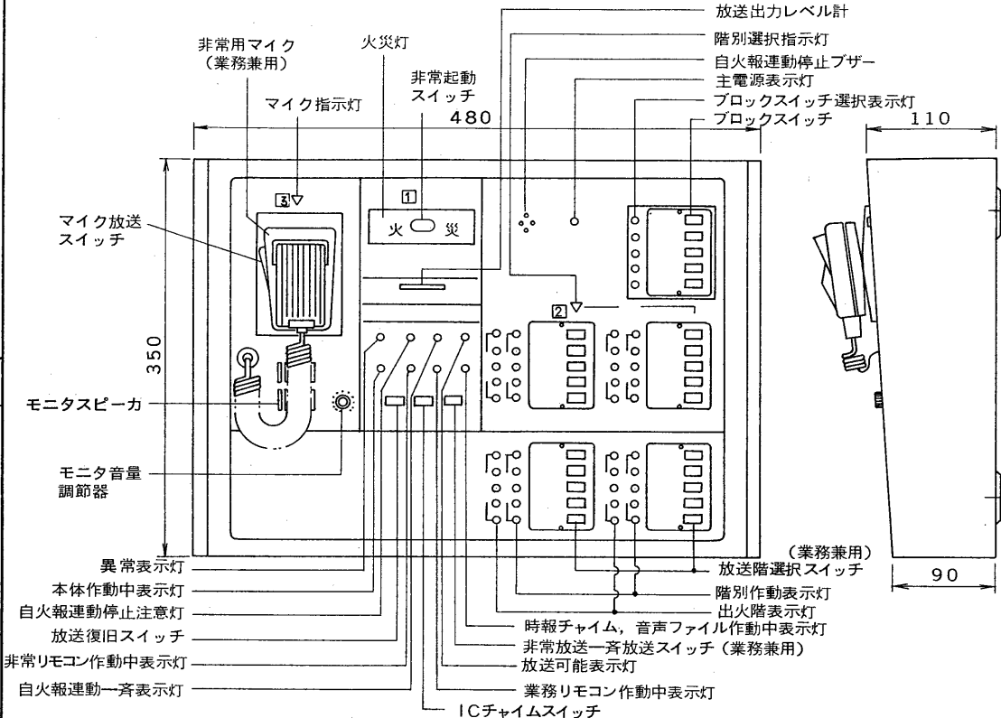
外觀寸法図
