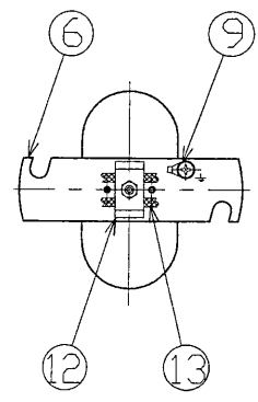
ソケット板下面図
