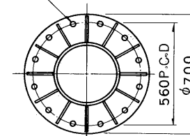
ベース部詳細
