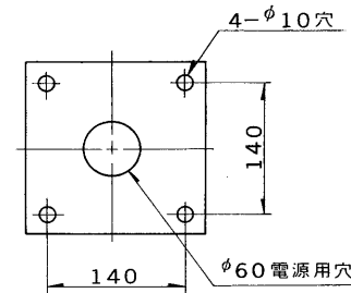
取付穴寸法
