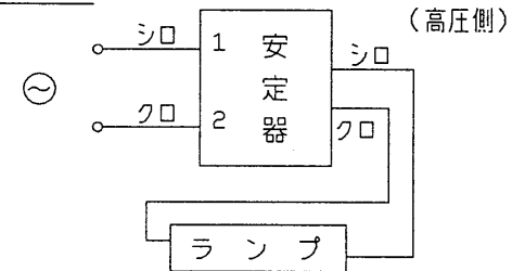
結線図
